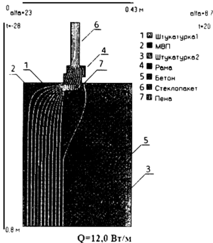
Рисунок Н.2 - Температурное поле узла конструкции, содержащего линейный элемент 1 Расчетный участок имеет размеры 426x800 мм. Площадь стены, вошедшей в расчетный участок, S_{1,1} = 0,532 \text{ м}^2 .
